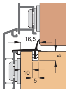
Einbauskizze 31122 (M 1:2)
