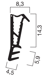
Profilquerschnitt 1028 (M 1:1)
