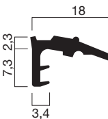
Profilquerschnitt 9022 (M 1:1)
