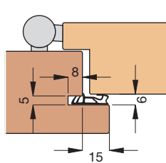
Einbauskizze 1008 (M 1:3)
