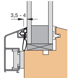
Einbauskizze 31171 (M 1:2)
