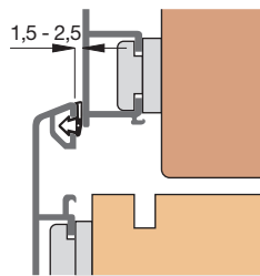
Einbauskizze 31279 (M 1:2)
