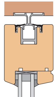
Einbauskizze 9020 (M 1:3)
