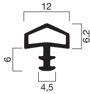
Profilquerschnitt 1004 (M 1:1)
