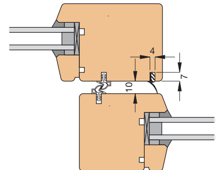
Einbauskeizze 9018 (1:3)
