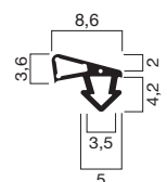
Profilquerschnitt 31279 (M 1:1)
