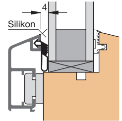
Einbauskizze 3183 (M 1:2)
