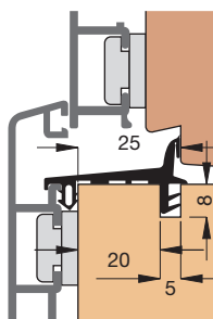
Einbauskizze 31168 (M 1:2)
