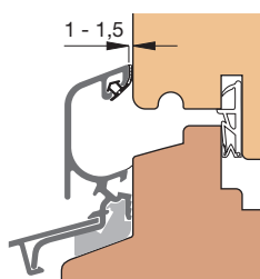
Einbauskizze 31151 (M 1:2)
