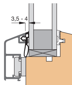
Einbauskizze 31171 (M 1:2)
