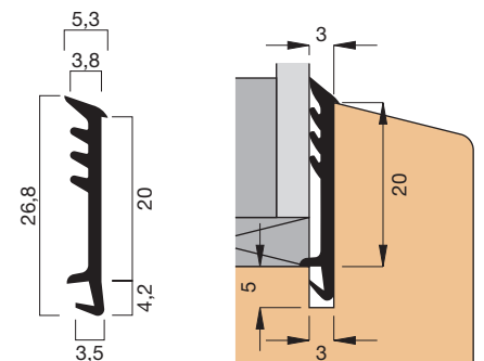
Profilquerschnitt 2912 (M 1:1)
