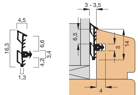
Profilquerschnitt 2911 (M 1:1)
