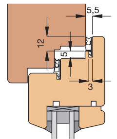
Einbauskizze 2058 im Überschlag (M 1:3)
