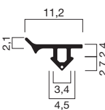
Profilquerschnitt 31335 (M 1:1)
