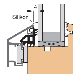
Einbauskizze 31320 (M 1:2)
