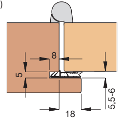
Einbauskizze 1046 (M 1:3)
