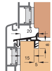
Einbauskizze 31190 (M 1:2)
