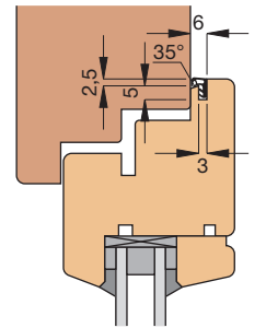
Einbauskizze 2611 (M 1:3)
