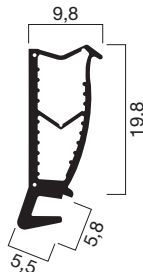
Profilquerschnitt 1042 (M 1:1)
