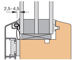
Einbauskizze 31397 (M 1:2)
