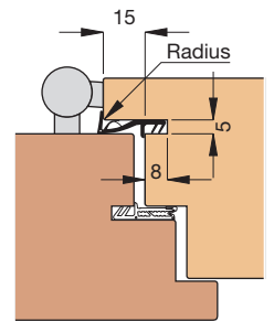
Einbauskizze 1030 (M 1:3)
