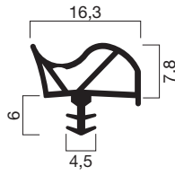
Profilquerschnitt 1027 (M 1:1)
