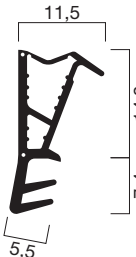
Profilquerschnitt 1038 (M 1:1)
