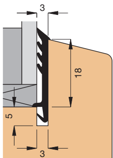
Einbauskizze 2914 (M 1:1)
