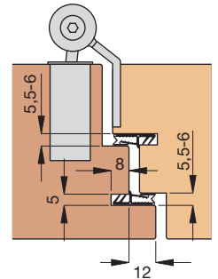
Einbauskizze 1044 (M 1:3)
