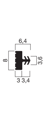
Profilquerschnitt 2928 (M 1:1)
