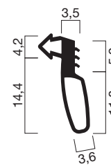
Profilquerschnitt 31125 (M 1:1)
