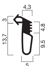
Profilquerschnitt 3183 (M 1:1)
