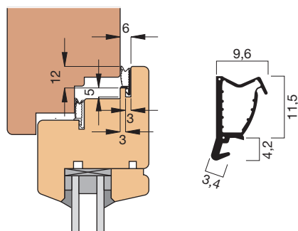
Einbauskizze 1041 im Überschlag (M 1:3) Profilquerschnitt 1041 (M 1:1)
