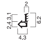
Profilquerschnitt 31317 (M 1:1)
