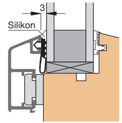
Einbauskizze 3146 (M 1:2)
