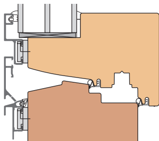
Einbauskizze 2064 (M 1:3)
