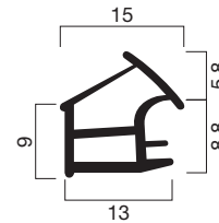
Profilquerschnitt 1603 (M 1:1)
