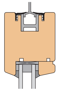
Einbauskizze 9012 (M 1:3)
