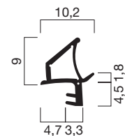
Profilquerschnitt 2063 (M 1:1)
