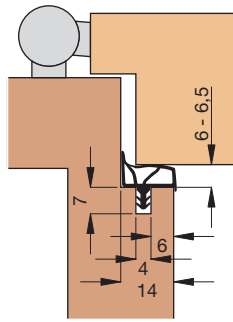
Einbauskizze 1027 (M 1:2)
