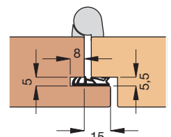
Einbauskizze 1021 (M 1:3)
