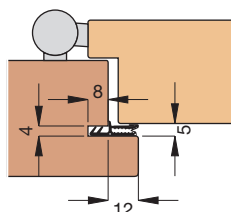
Einbauskizze 1036 (M 1:3)
