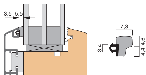
Einbauskizze 31231 (M 1:2)
