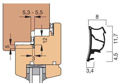
Einbauskizze 2054 im Flügelfalz (M 1:3) Profilquerschnitt 2054 (M 1:1)
