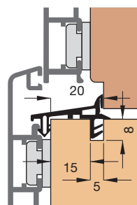
Einbauskizze 31190 (M 1:2)
