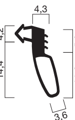
Profilquerschnitt 31197 (M 1:1)
