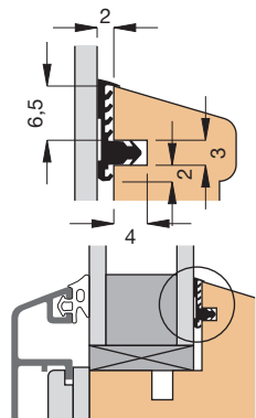
Einbauskizze 2906 (M 1:1 / M 1:2)
