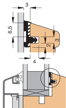
Einbauskizze 2907 (M 1:1 / M 1:2)
