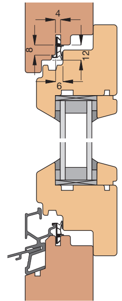
Einbauskizze 2041 (M 1:3)
