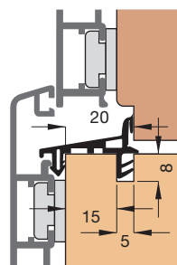
Einbauskizze 3194 (M 1:2)
