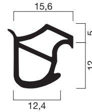
Profilquerschnitt 1601 (M 1:1)
