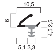
Profilquerschnitt 2059 (M 1:1)
