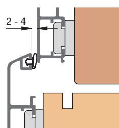
Einbauskizze 3153 (M 1:2)
