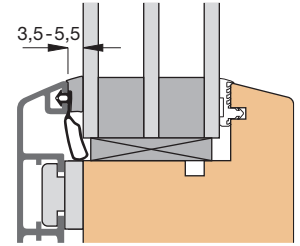
Einbauskizze 31228 (M 1:2)
