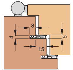
Einbauskizze 1037 (M 1:3)
