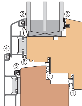
Einbauskizze eines Gesamtsystems für ein Holz-/Aluminiumfenster (M 1:3)
