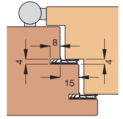
Einbauskizze 1028 (M 1:3)
