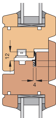
Einbauskizze 2044 (M 1:3)
