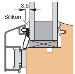
Einbauskizze 31125 (M 1:2)
