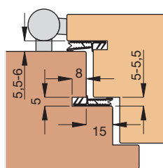
Einbauskizze 1017 (M 1:3)
