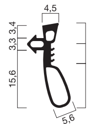
Profilquerschnitt 31171 (M 1:1)
