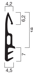
Profilquerschnitt 2032 (M 1:1)
