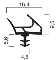
Profilquerschnitt 1035 (M 1:1)
