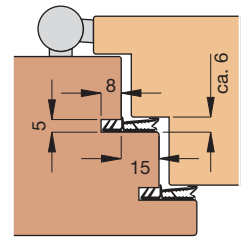
Einbauskizze 1038 (M 1:3)
