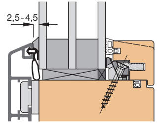
Einbauskizze Fixverglasung 31397 (M 1:2)
