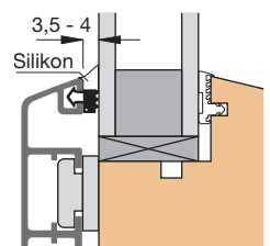
Einbauskizze 31264 (M 1:2)
