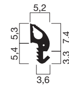
Profilquerschnitt 31287 (M 1:1)
