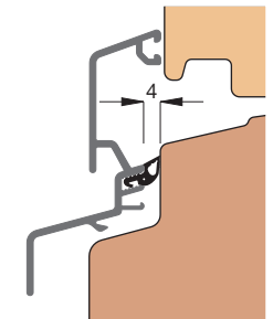
Einbauskizze 31287 (M 1:2)
