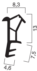
Profilquerschnitt 2030 (M 1:1)
