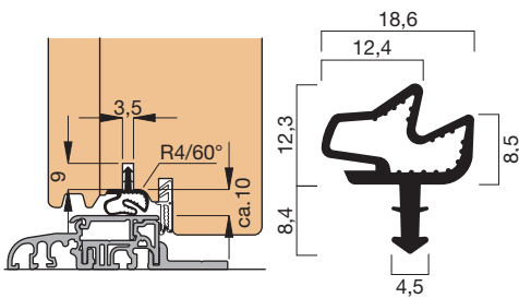
Einbauskizze 1033 (M 1:3)
