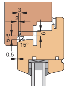
Einbauskizze 2063 (M 1:3)
