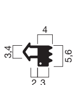
Profilquerschnitt 31264 (M 1:1)
