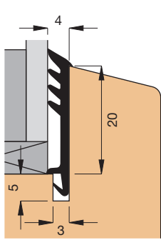
Einbauskizze 2913 (M 1:1)
