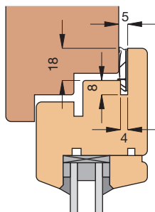
Einbauskizze 2621 (M 1:3)
