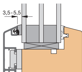
Einbauskizze 31211 (M 1:2)
