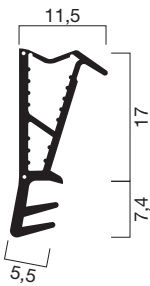
Profilquerschnitt 1032 (M 1:1)
