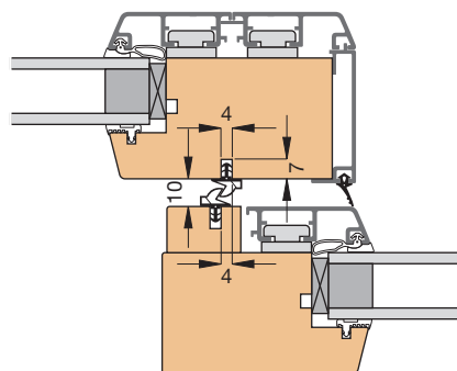
Einbauskeizze 9014 und 9015 (1:3)
