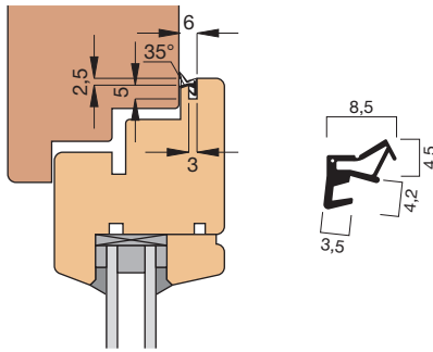
Einbauskizze 2622 (M 1:3)
