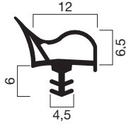
Profilquerschnitt 1019 (M 1:1)
