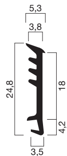
Profilquerschnitt 2914 (M 1:1)
