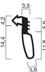
Profilquerschnitt 31125 (M 1:1)
