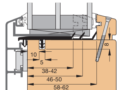
Einbauskizze 31300 (M 1:2)
