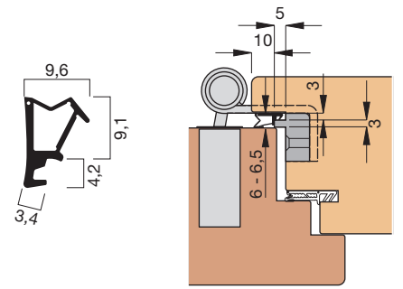
Profilquerschnitt 1039 (M 1:1)
