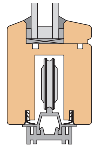
Einbauskizze 9007 (M 1:3)
