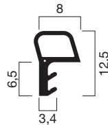
Profilquerschnitt 9025 (M 1:1)
