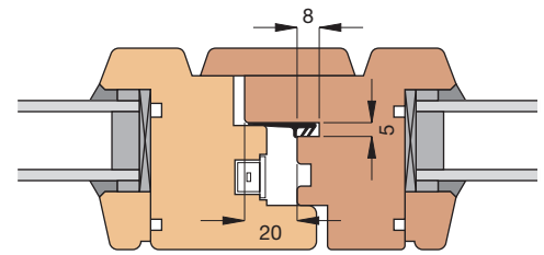
Einbauskizze 2047 (M 1:3)
