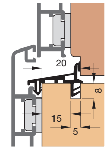
Einbauskizze 3194 (M 1:2)
