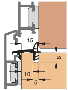
Einbauskizze 3156 (M 1:2)
