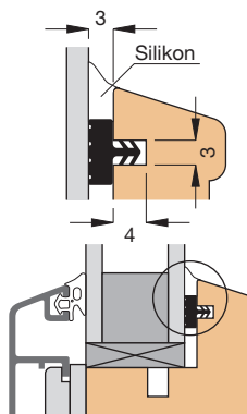
Einbauskizze 2928 (M 1:1)
