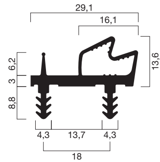
Profilquerschnitt 13110 (M 1:1)
