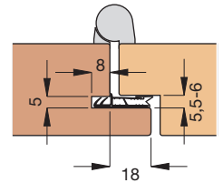
Einbauskizze 1046 (M 1:3)
