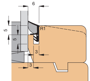
Profilquerschnitt 2807 (M 1:1)
