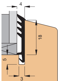
Einbauskizze 2915 (M 1:1)
