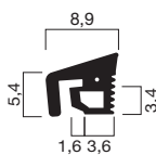
Profilquerschnitt 31285 (M 1:1)
