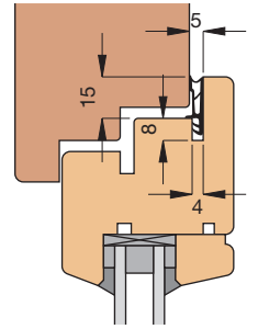
Einbauskizze 2603 (M 1:3)
