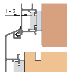
Einbauskizze 31335 (M 1:2)
