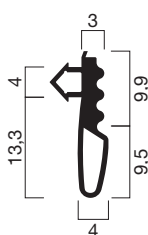
Profilquerschnitt 3146 (M 1:1)
