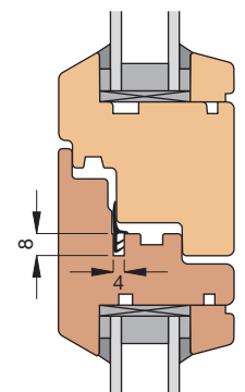
Einbauskizze 2061 (M 1:3)
