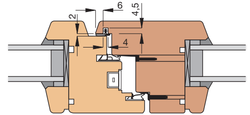
Einbauskizze 2057 (M 1:3)
