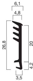
Profilquerschnitt 2913 (M 1:1)
