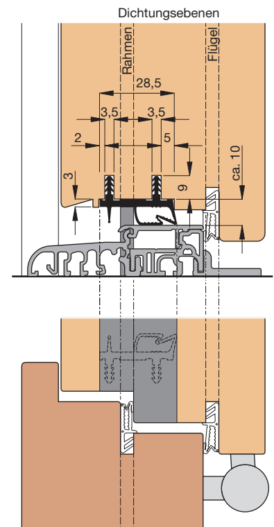
Einbauskizze 13110 (M 1:2)
