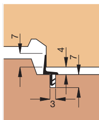
Einbauskizze 2065 (M 1:2)
