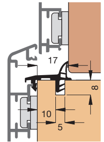
Einbauskizze 31123 (M 1:2)
