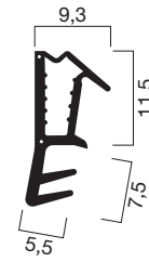
Profilquerschnitt 1044 (M 1:1)
