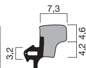
Profilquerschnitt 31271 (M 1:1)
