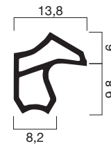
Profilquerschnitt 1602 (M 1:1)
