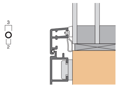
Profilquerschnitt 31395 (M 1:1)
