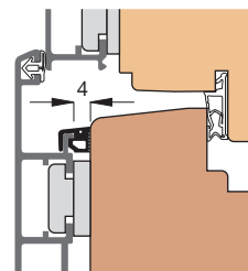
Einbauskizze 31285 (M 1:2)
