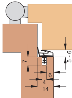
Einbauskizze 1035 (M 1:2)
