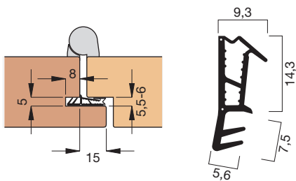
Profilquerschnitt 1045 (M 1:1)
