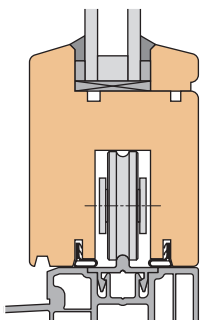
Einbauskizze 9025 (M 1:3)
