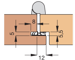
Einbauskizze 1020 (M 1:3)
