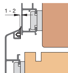
Einbauskizze 31335 (M 1:2)
