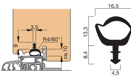
Einbauskizze 1040 (M 1:3)
