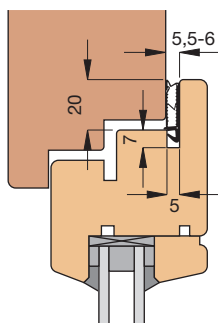
Einbauskizze 1042 (M 1:3)
