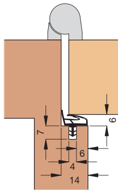
Einbauskizze 1035 (M 1:2)
