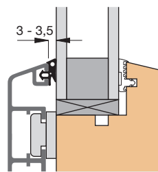
Einbauskizze 31105 (M 1:2)
