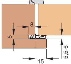
Einbauskizze 1045 (M 1:3)
