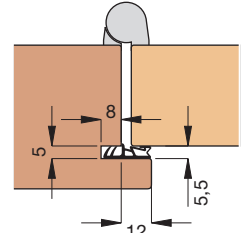
Einbauskizze 1020 (M 1:3)
