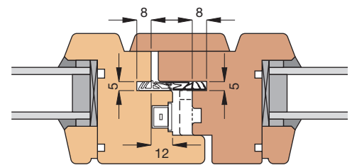
Einbauskizze 2202/2201 (M 1:3)
