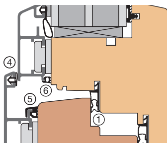
Einbauskizze eines Gesamtsystems für ein Holz-/Aluminiumfenster (M 1:3) 1 - 1 Dichtung für Flügelfalz und Überschlag (AFK2054) 2 - Trockenverglasung für außen (z.B. SGFK31207) 3 - Trockenverglasung für innen (z.B. AA2907) 4 - Anschlagdichtung (z.B. FF2048) 5 - Fugenabschlussdichtung (z.B. AF31263) 6 - Anschlussdichtung (z.B. A 31106)
