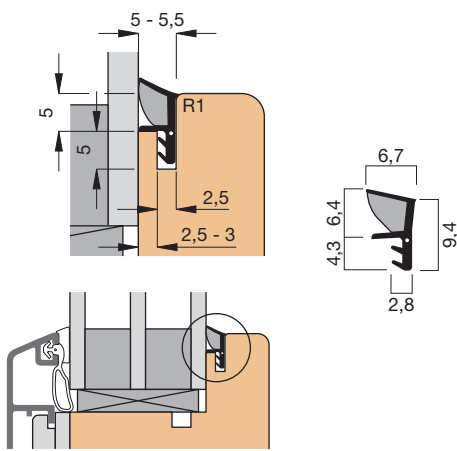
Einbauskizze 2806 (M 1:1 / M 1:2)
