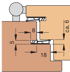
Einbauskizze 1032 (M 1:3)
