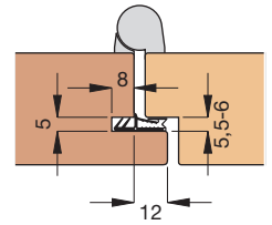
Einbauskizze 1044 (M 1:3)
