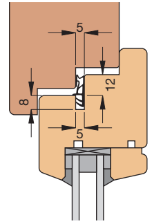
Einbauskizze 2003 (M 1:3)
