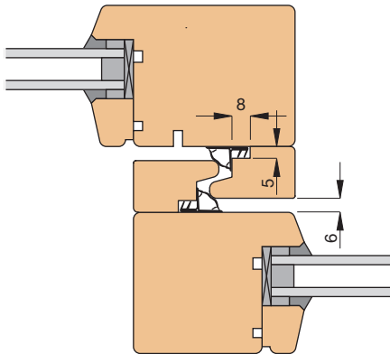
Einbauskizze unterer Anschluss 9024 (M 1:3)
