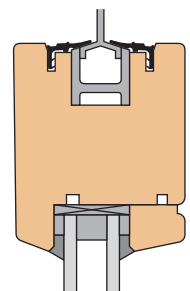
Einbauskizze 9022 (M 1:3)
