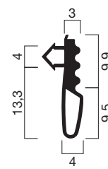
Profilquerschnitt 3146 (M 1:1)
