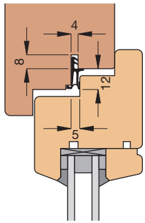
Einbauskizze 2024 (M 1:3)
