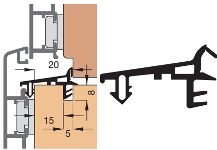
Einbauskizze 31190 (M 1:2)
