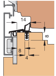
Einbauskizze 31316 (M 1:2)
