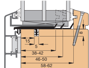
Einbauskizze 31299 (M 1:2)
