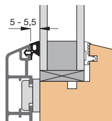
Einbauskizze 31169 (M 1:2)
