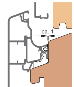
Einbauskizze 31317 (M 1:2)
