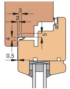
Einbauskizze 2059 (M 1:3)
