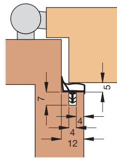
Einbauskizze 1019 (M 1:2)
