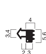
Profilquerschnitt 31264 (M 1:1)
