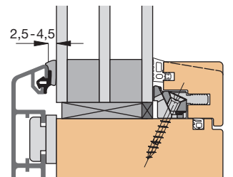
Einbauskizze Fixverglasung 31270 (M 1:2)
