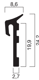
Profilquerschnitt 2060 (M 1:1)
