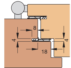
Einbauskizze 1029 (M 1:3)
