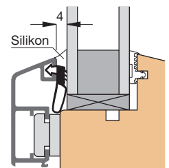
Einbauskizze 31197 (M 1:2)
