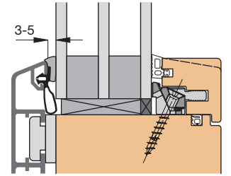
Einbauskizze Fixverglasung 31267 (M 1:2)
