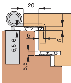
Einbauskizze 1042 (M 1:3)
