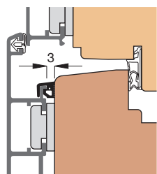
Einbauskizze 31263 (M 1:2)
