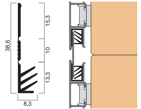
Profilquerschnitt 31131 (M 1:1)
