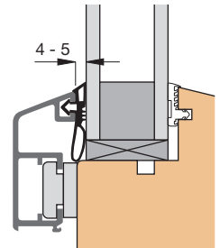
Einbauskizze 3198 (M 1:2)
