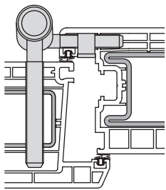
Einbauskizze 3529 (M 1:3)
