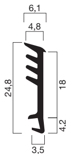
Profilquerschnitt 2915 (M 1:1)
