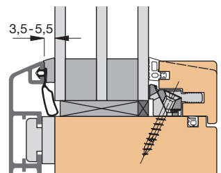
Einbauskizze Fixverglasung 31228 (M 1:2)
