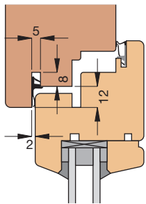
Einbauskizze 2043 (M 1:3)
