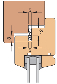
Einbauskizze 2001 (M 1:3)
