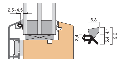
Einbauskizze 31400 (M 1:2)
