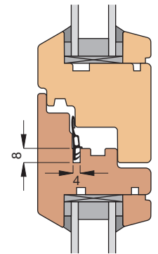
Einbauskizze 2032 (M 1:3)
