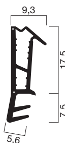
Profilquerschnitt 1046 (M 1:1)
